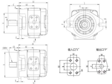
替换 VOITH 油泵参数 Replace the Parameters of VOITH Oil Pump
